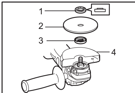
► 1. Contratuercas 2. Disco de corte abrasivo / Disco de diamante 3. Brida interior 4. Protector de disco para disco de corte abrasivo / disco de diamante
