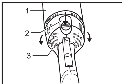
► 1. Boîtier du moteur 2. Bouton de verrouillage 3. Manche
